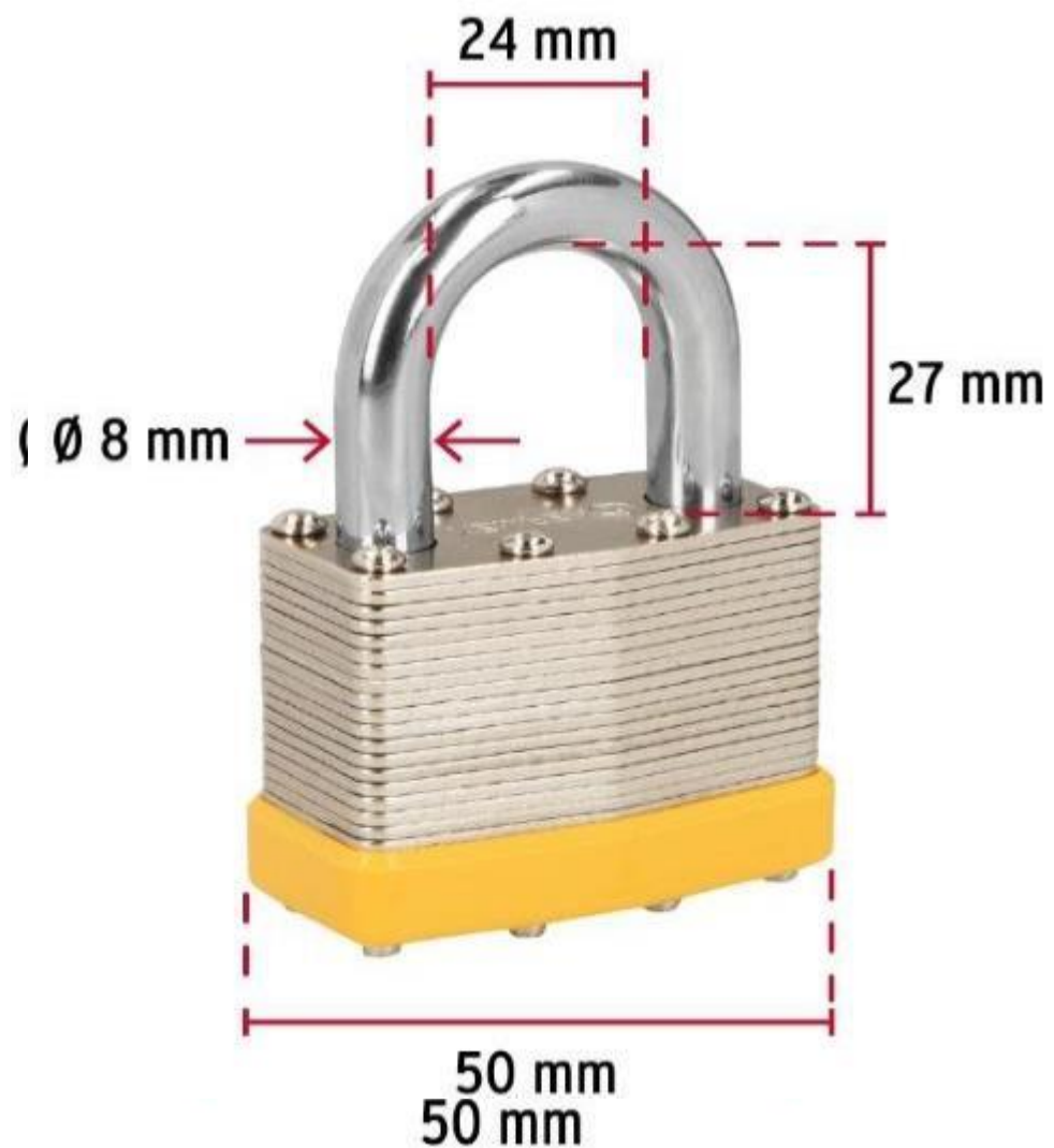
CANDADO PARA LAMINADO 30-40-50-60
